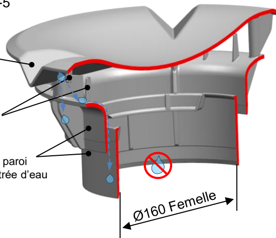
VX16A en coupe
